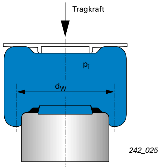
Schlauchrollbalg
